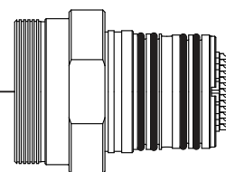
Kabelverlängerung für rückseitigen Öldruck cable connecting receptacle for rearside oil pressure
