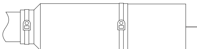
Endgehäuse mit FVMQ-Formteil und Titan-Schellenbändern moulding endbell with FVMQ boot and titanium clamps
